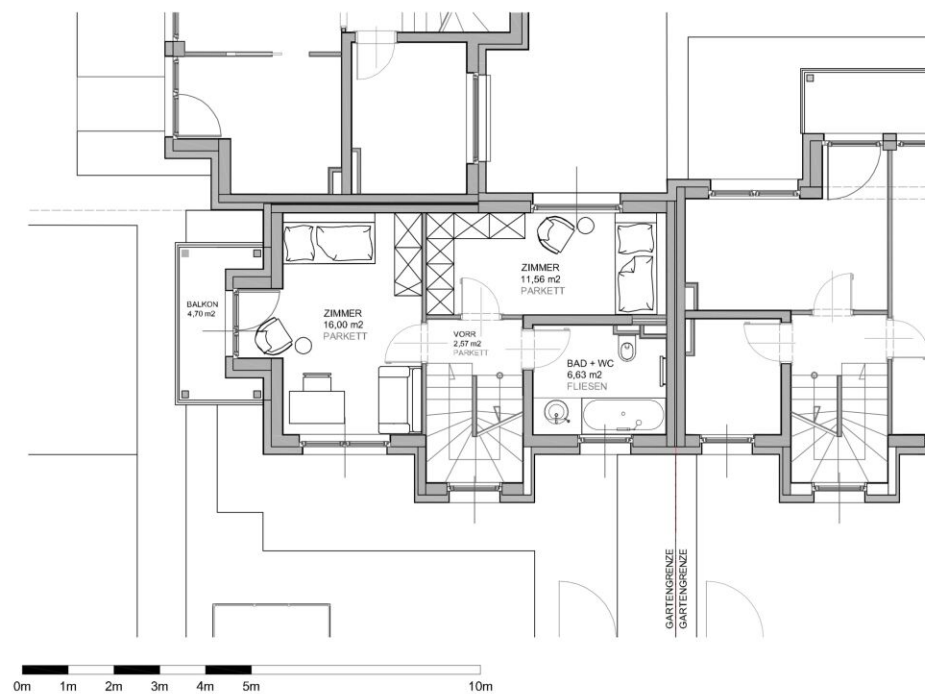
OBERGESCHOSS
