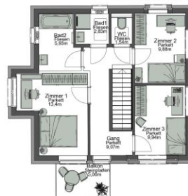
1.OBERGESCHOSS
